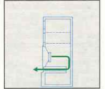
Weg der rückwärtigen Schallenergie durch den Transmissionline-Tonkanal.
