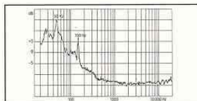
Wiedergabe-Fremdspannung mit herkömmlichem Trafo.
