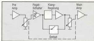
Rauschminimierung durch doppelte Lautstärkeregelung.
